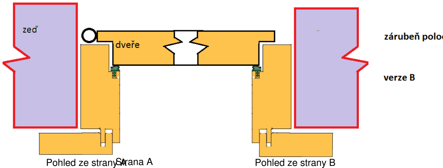
Příklady nové zárubně verze B
