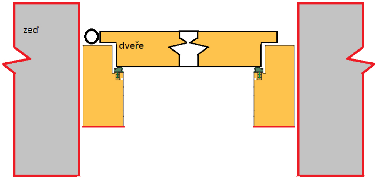
Přehledová zárubeň
