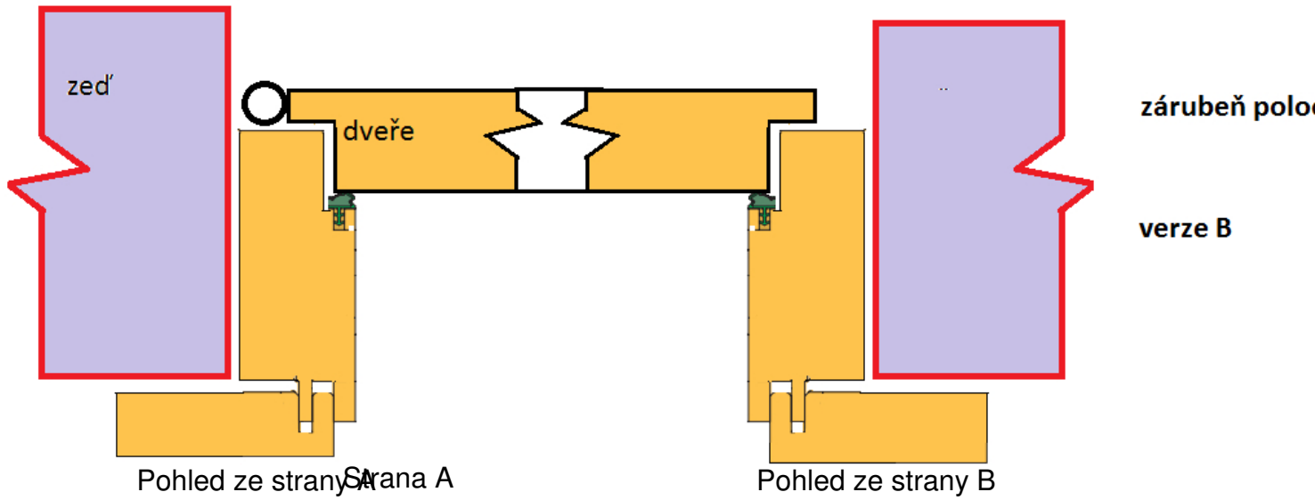
Příkladová zárubeň verze B
